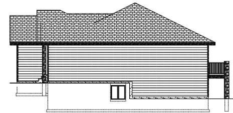
RIGHT ELEVATION SCALE: 1/8" = 1'-0"
